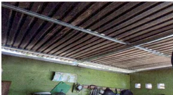
Foto 7: Sustitución de estructura de soporte de madera por metal
